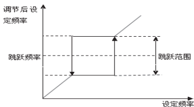
图 F2-5 跳跃频率设定图
