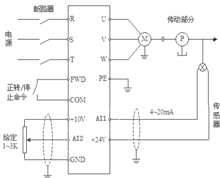
图 F8-1 模拟反馈控制系统示意图
