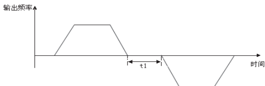
图 F2-6 正反转死区时间示意图
