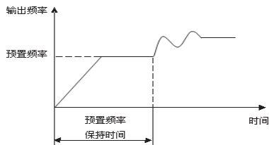
图 F8-3 闭环预置频率运行示意图
