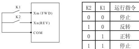
图 F6-1 二线式控制模式 1 示意图
