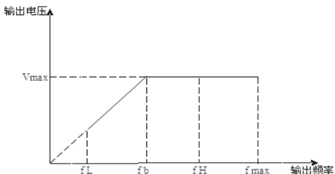
图 F1-1 电压与频率示意图
