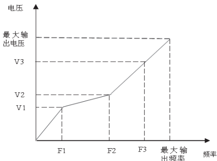
图 F3-3 用户设定 V/F 曲线示意图
