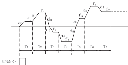
图 F9-4 简易 PLC 运行示意图
