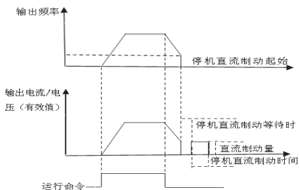
图 F2-3 停机直流制动示意图
