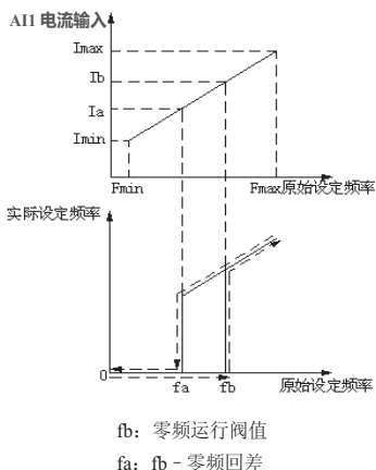
图 F7-2 零频功能示意图
