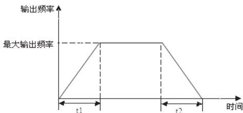
图 F1-2 加速时间和减速时间示意图
