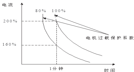
图 FA-1 电机过载保护曲线示意图
