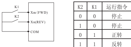
图 F6-2 二线式控制模式 2 示意图
