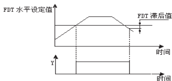
图 F6-6 频率水平检测示意图
