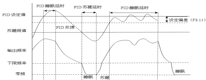
图 F8-4 睡眠与苏醒功能示意图
