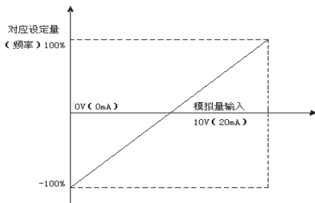
图 F7-1 输入模拟量与频率关系对应示意图
