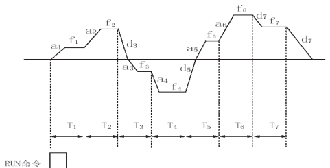
图 F9-2 PLC 单循环示意图
