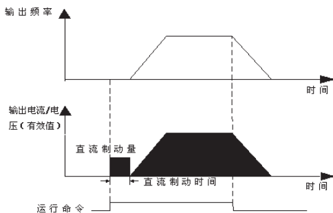
图 F2-2 起动直流制动示意图
