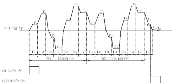
图 F9-3 PLC 连续示意图
