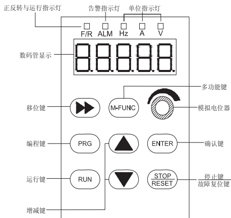
图1 LED操作面板示意图
