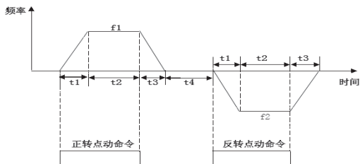
F2-4 点动运行图
