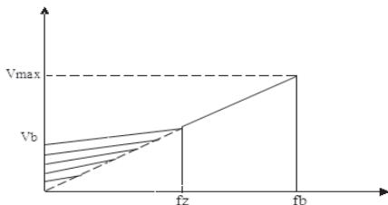
图 F3-2 转矩提升示意图
