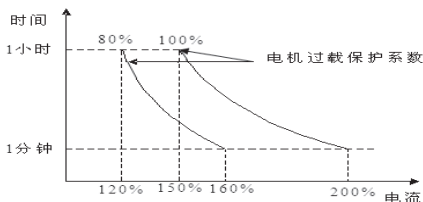
图 FA-2 电机过载保护系数设定示意图
