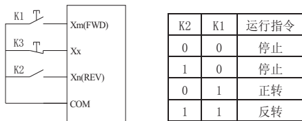
图 F6-4 三线式控制模式 2 示意图
