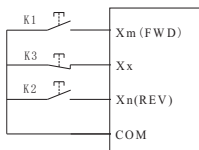
图 F6-3 三线式控制模式 1 示意图
