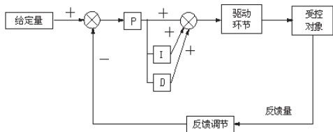
图 F8-2 PID 调节示意图
